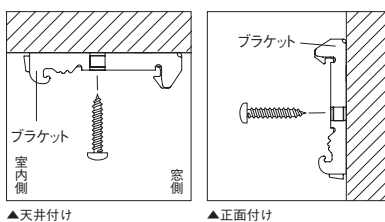
▲天井付け
