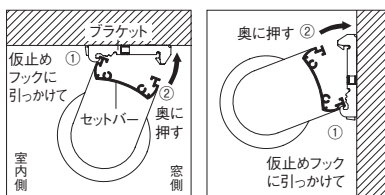
▲天井付け
